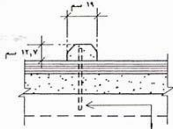
قضبان من حديد تسليح مغروسان عمودياً لتثبيت المصددة بالأرض (العدد ١٢٢ و ١)
