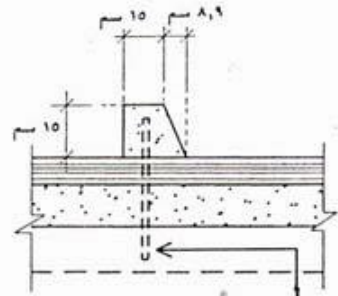
قضبان من حديد تسليح مغروسان عمودياً لتثبيت المصددة بالأرض (العدد ١٢٢ و ١)
